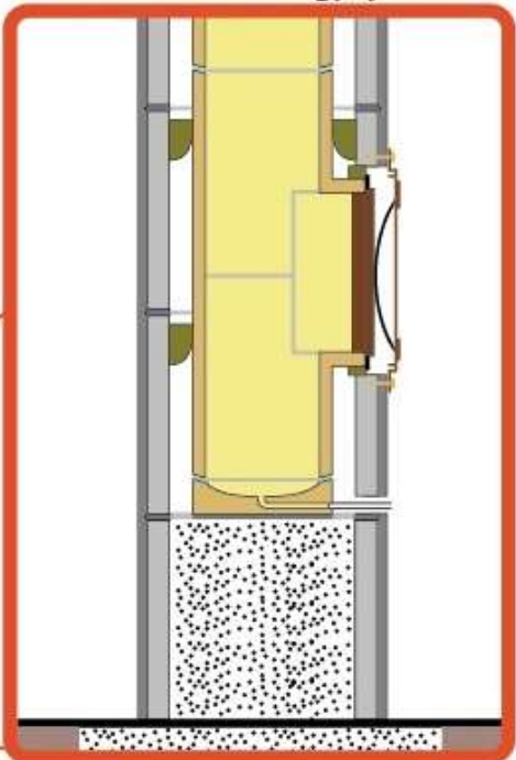
Kettős záródású koromzsákajtó és kondenzvíz gyűjtő
