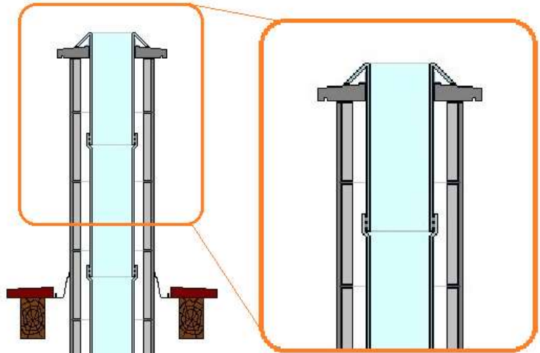
Beton kéményfedkő, saválló acél kéménykúp
