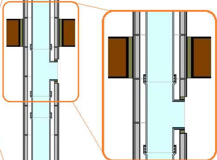
Födémátvezetés dilatációval és bekötőidom
