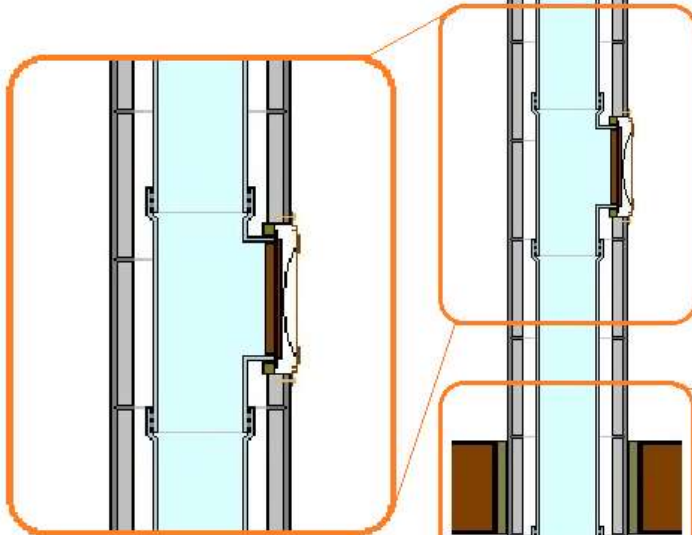
Kettős záródású felső tisztítóajtó
